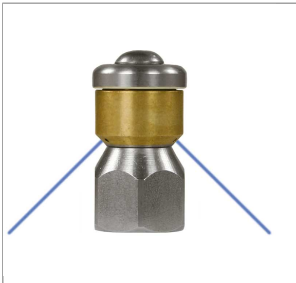
Suttner Rotations-Rohrreinigungsdüse ST-49.1
