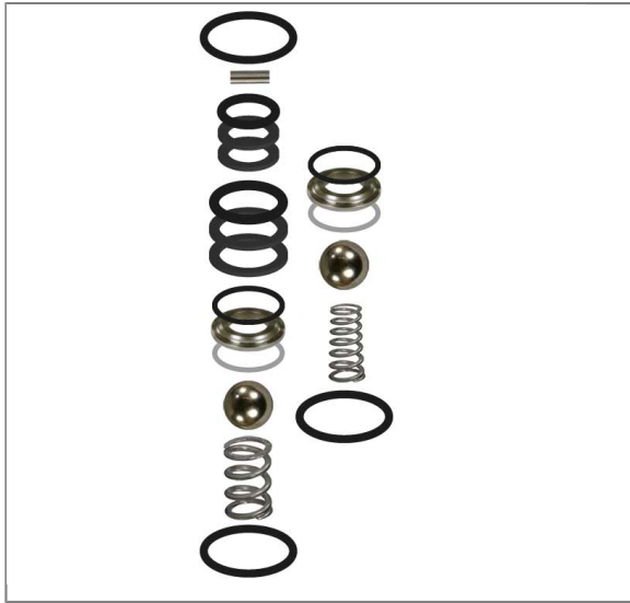
Rep.Kit ST-250 und UL250 Kugelrückschlagventil
