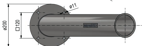
Montage simple : La plaque de montage est pourvue de quatre trous de Ø 11 mm.
