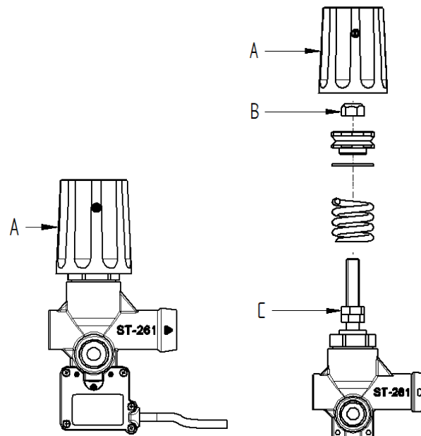
Figure 1 A - Einstellrad
